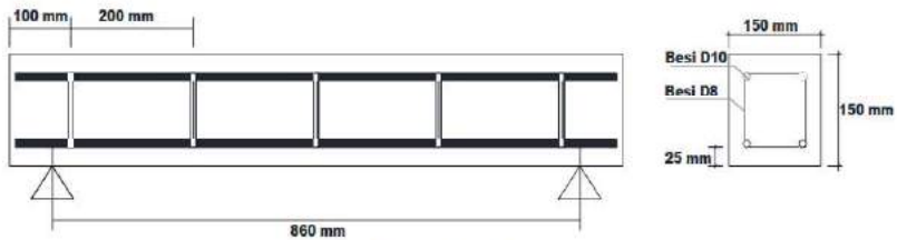
Gambar 5. Balok uji beton bertulang baja
