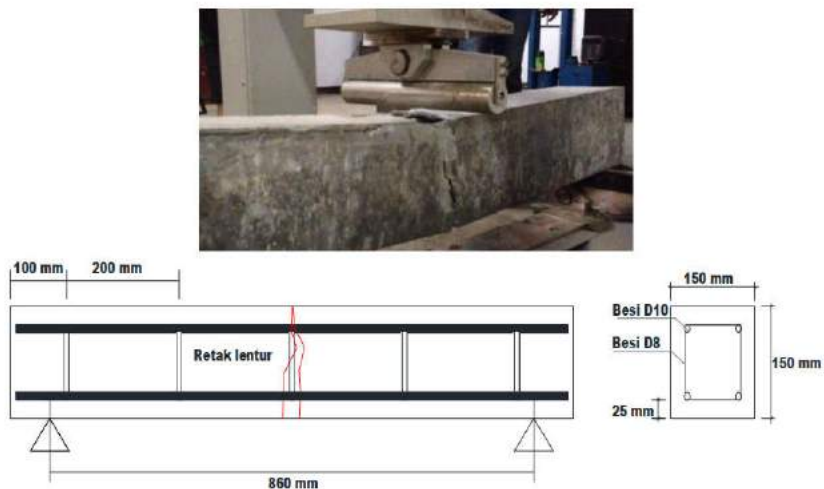
Gambar 6. Pola retak pada balok kontrol
