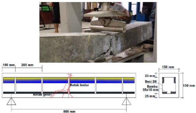
Gambar 8. Pola retak balok tipe 2
