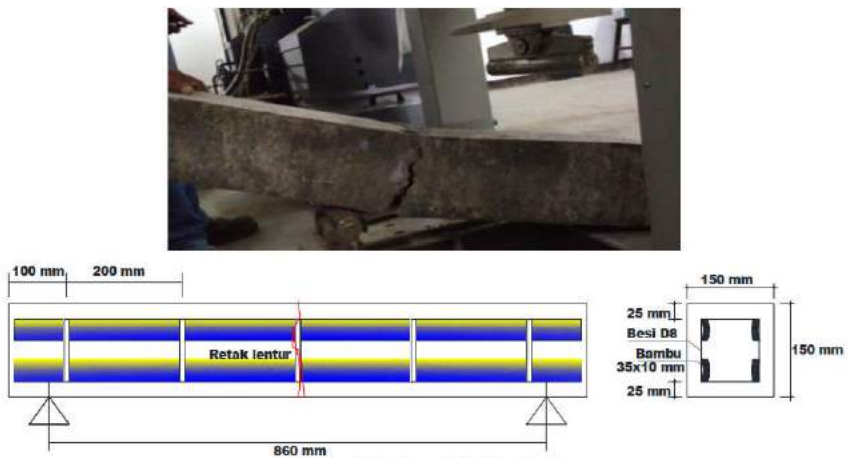
Gambar 7. Pola retak balok tipe 1
