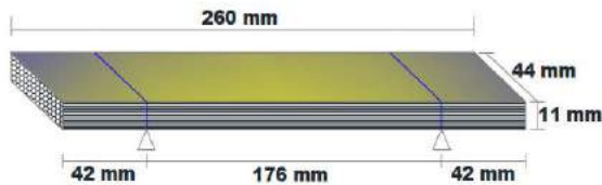
Gambar 3. Spesimen uji lentur bamboo
