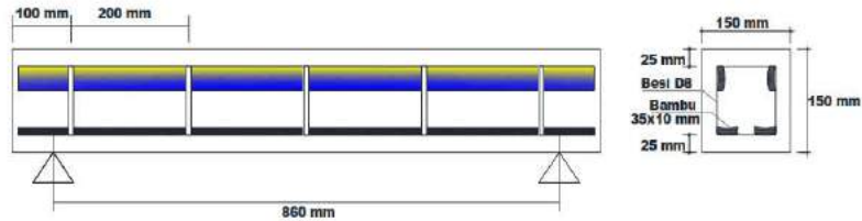
Gambar 4. Balok uji beton bertulang bambu
