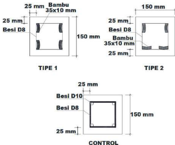
Gambar 1. Susunan tulangan pada penampang balok
