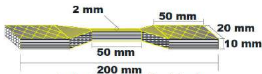
Gambar 2. Spesimen uji tarik bamboo
